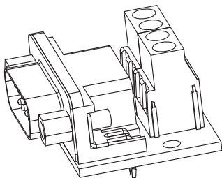
9PIN转4PIN转接器 ADP-090401 (232、485与422专用, 需另行订购)
