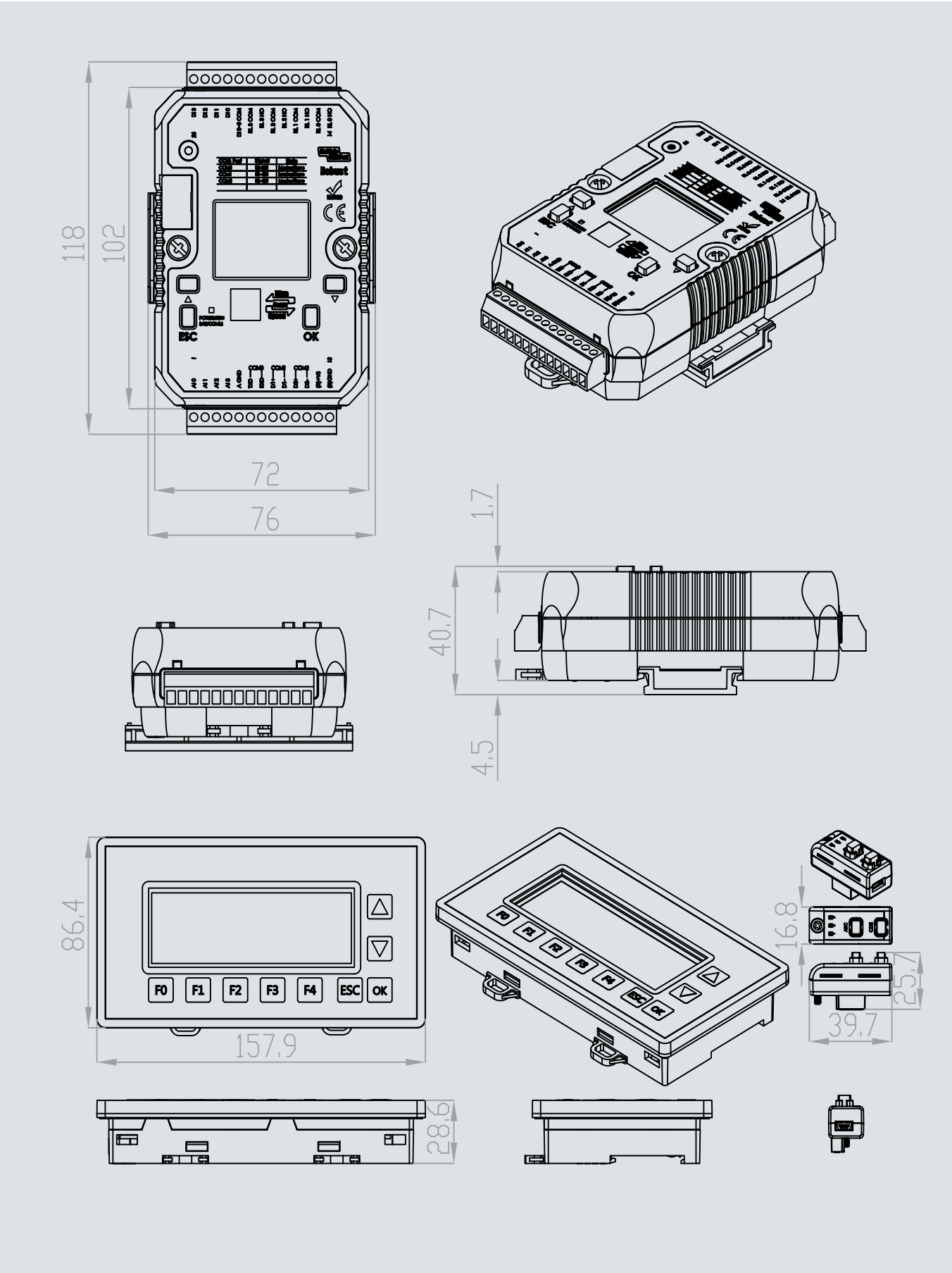
外觀尺寸
